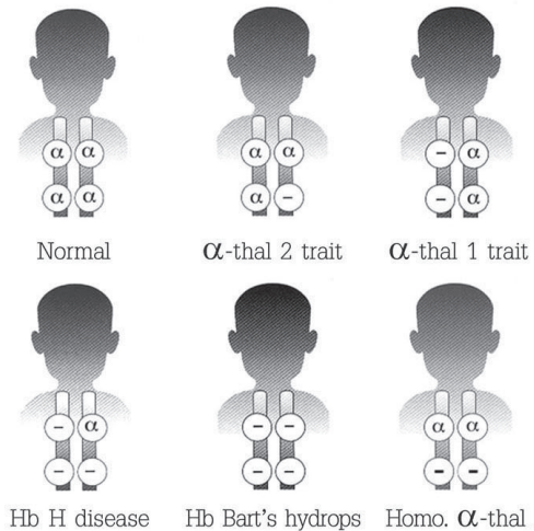
รูปที่ 3 แสดงแอลฟายีนใน คนปกติ พาหะแอลฟาธาลัสซีเมีย 2 พาหะแอลฟาธาลัสซีเมีย 1 โรคฮีโมโกลบินเอช ฮีโมโกลบินบาร์ทซ์ไฮดรอป และ ไฮโปซีทิกธาลัสซีเมีย 2 ตามลำดับ
