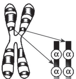
รูปที่ 2 แสดงแอลฟายีนซึ่งอยู่บนโครโมโซมคู่ที่ 16
