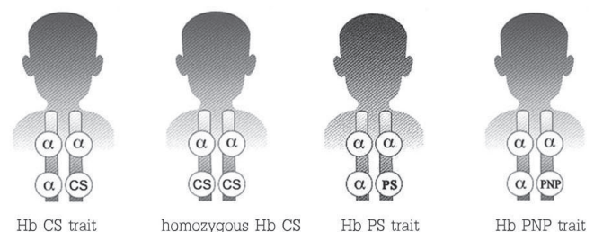
รูปที่ 4 แสดงแอลฟายีนชนิด non-deletion ในพาหะฮีโมโกลบินคอนสแตนต์สปริง ไฮโปซีทิกธาลัสซีเมียชนิดคอนสแตนต์สปริง ฮีโมโกลบินปากเซ และฮีโมโกลบินปากน้ำโพ ตามลำดับ
